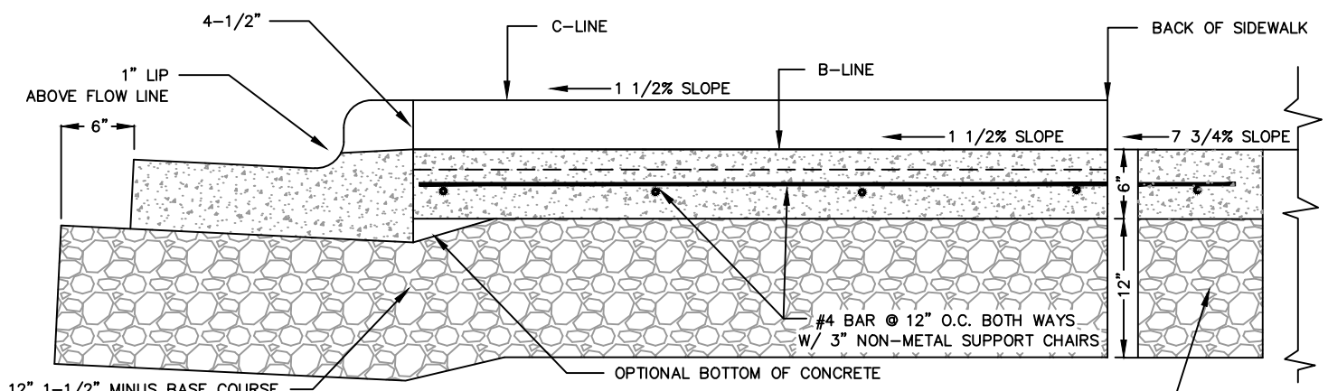
SECTION A-A
